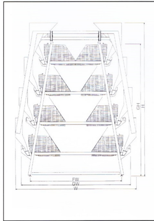
育成A型 COMFORT ビットスクレーパー 又は、糞ベルト
