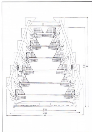
集約の PLASTICA 糞乾エアーダクト ベルトケージ
