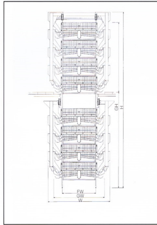
中間作業台付 PLASTICA
